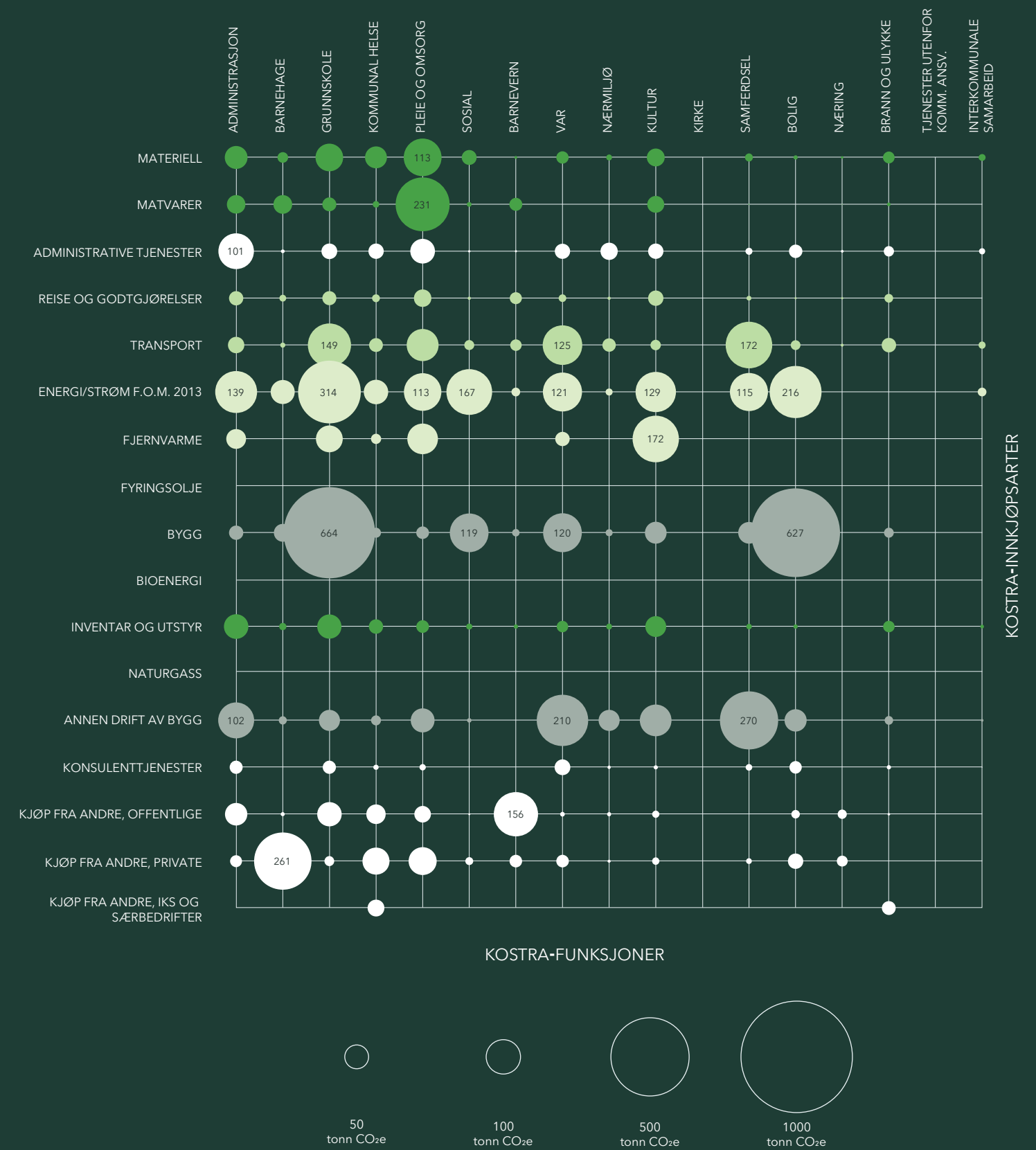
Figur 5: Klimafotavtrykk for Alstahaug kommune i år 2020, detaljert nivå, tall i tonn CO 2 e
