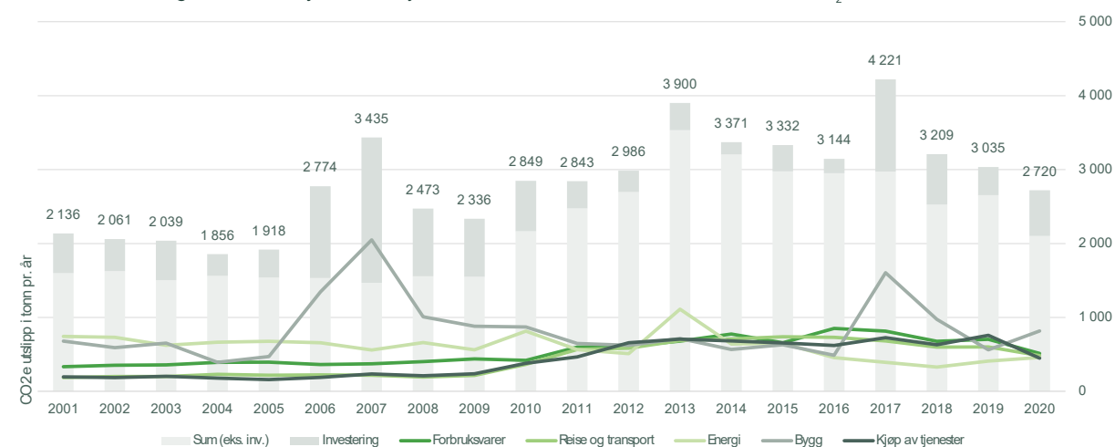
Figur 18: Utvikling i klimafotavtrykk for Leirfjord kommune fra år 2001 til 2020, tall i tonn CO 2 e
