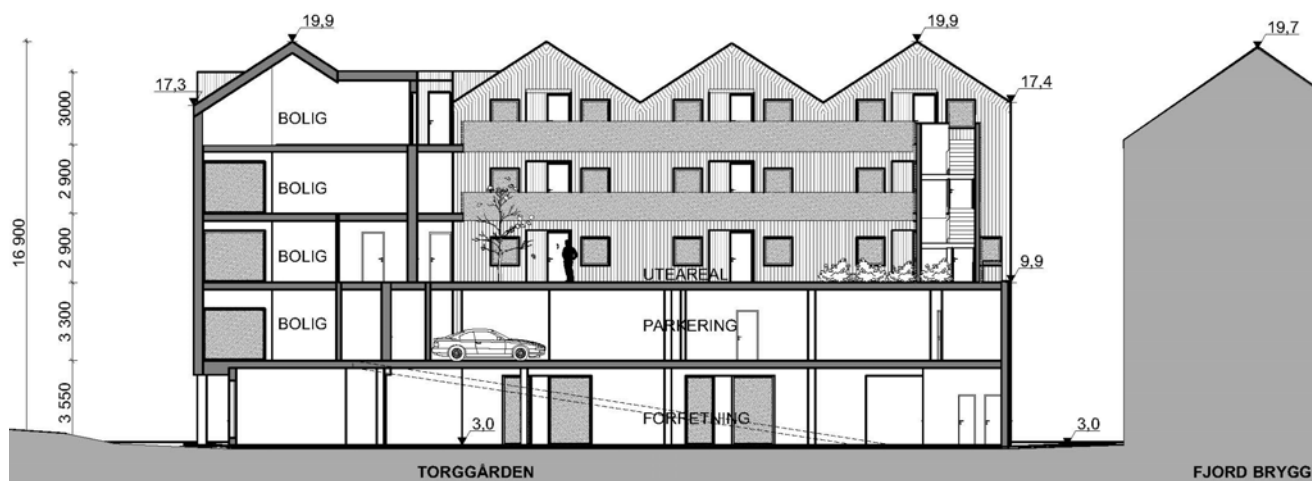
Snitt som viser høyder
