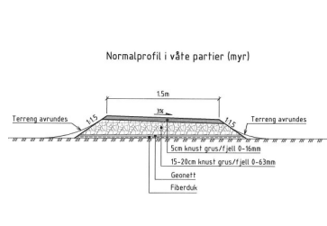
Figur 12: Prinsipp for opprusting av hovedstien over Åsen.
